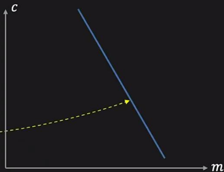
Parameter Space
